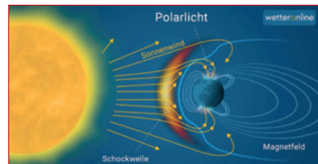
So entsteht das Polarlicht. Quelle: wetteronline.at
