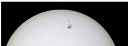
Großer Sonnenfleck, Weißlichtaufnahme. Foto: Manfred Fischer
